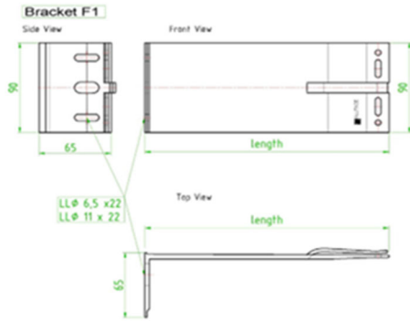
Diagram 1 - Bracket F1
